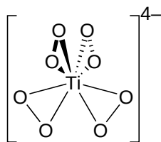
图 18: [\text{Ti}(\text{O}_2)_4]^{4-} 的结构
