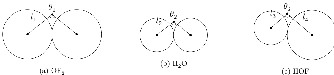
图 17: \text{OF}_2 , \text{H}_2\text{O} 和 \text{HOF} 的 LCP 模型示意图
