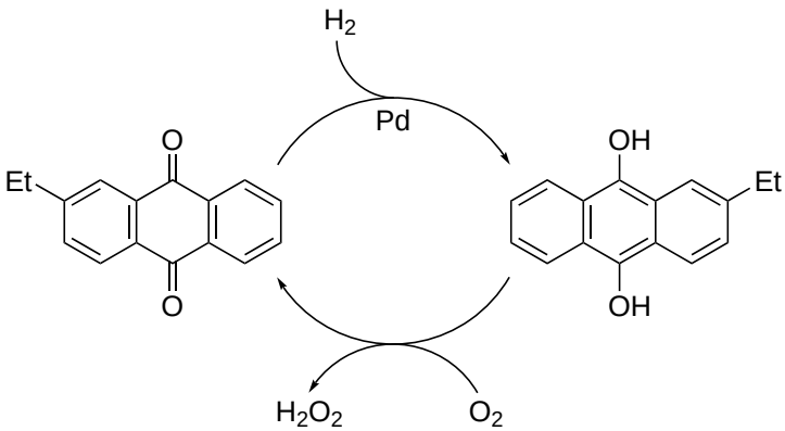
图 16: 乙基蒽醌法制备 H 2 O 2
