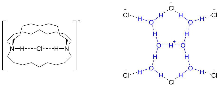
图 11: [(\text{C}_9\text{H}_{18})_3(\text{NH})_2\text{Cl}]^+ 和 \text{H}_{13}\text{O}_6^+ 的结构
