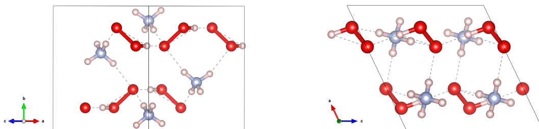
(a) \text{NH}_4\text{OOH} 沿 \vec{a} + \vec{c} 方向的投影图
